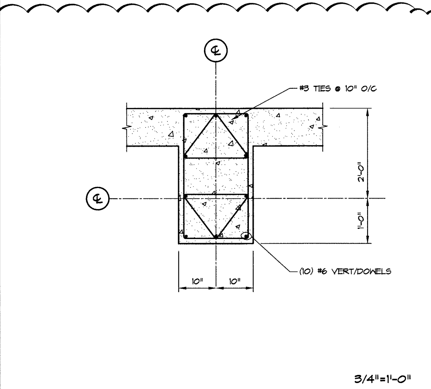
6 PIER P6
